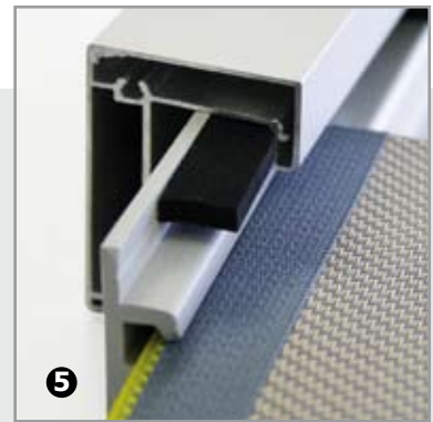
DETAIL GELEIDINGSSYSTEEM
